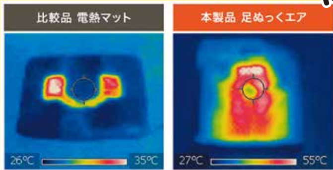
市販の電熱マットとの比較(使用開始直後)では、広範囲に温風が広がり、あっという間に55度に。
